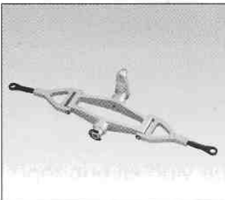
50PV0097 Alu Nickansteuerung
